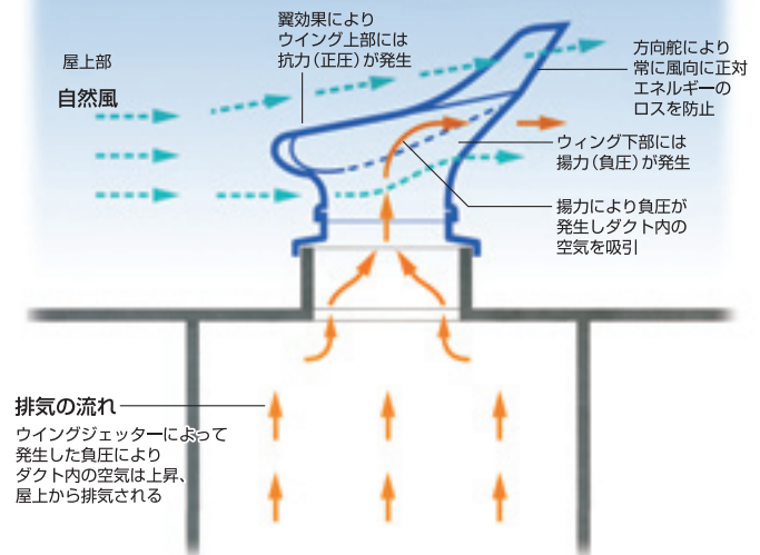
ウイングジェッターシステム概念図
