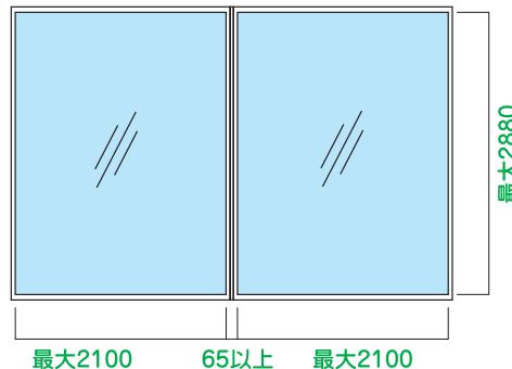
耐熱強化ガラス入 FIX 連窓 国土交通大臣個別認定番号 EA-0207
