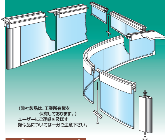
免震用壁面方立・MT500/530 ・MT800/830 * /寸法は切断可能
